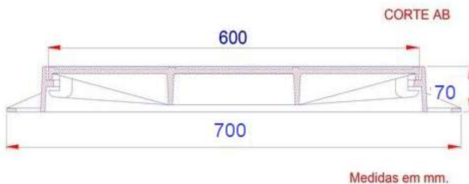
Figura 1. Layout com medidas MÍNIMAS.
